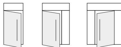
Porte 1 vantail et imposte Porte avec fixe et imposte Porte avec 2 fixes et imposte
